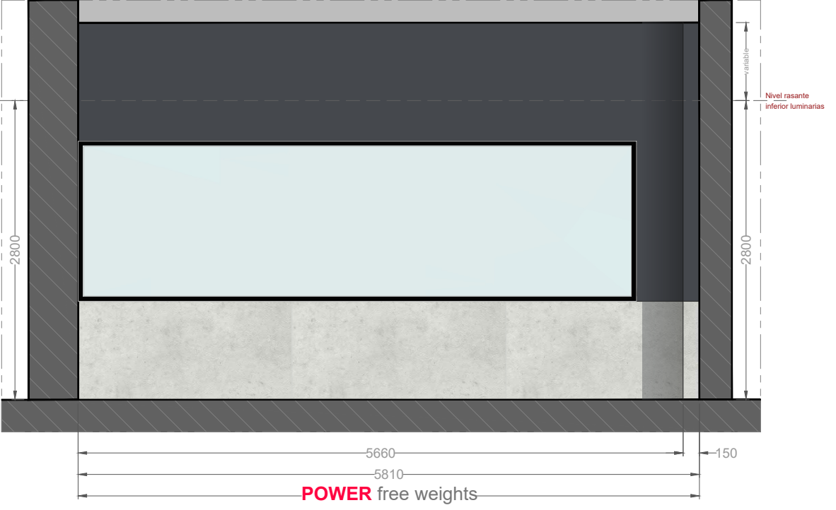
Alzado N | E: 1/50
