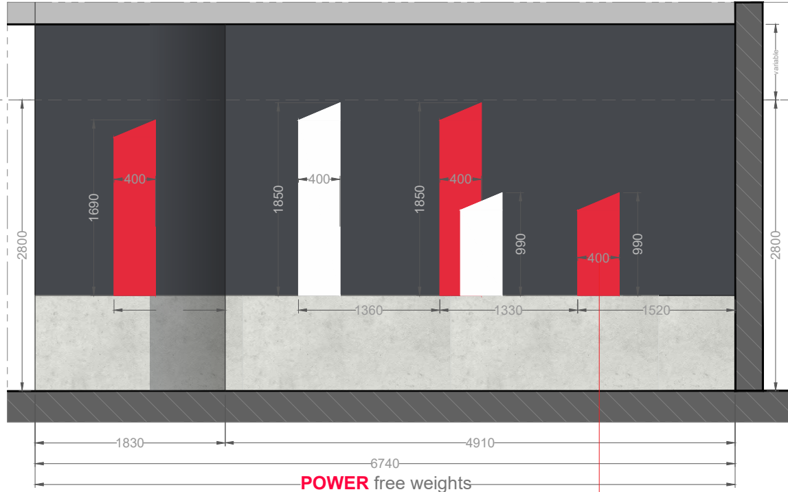
Alzado I | E: 1/50
