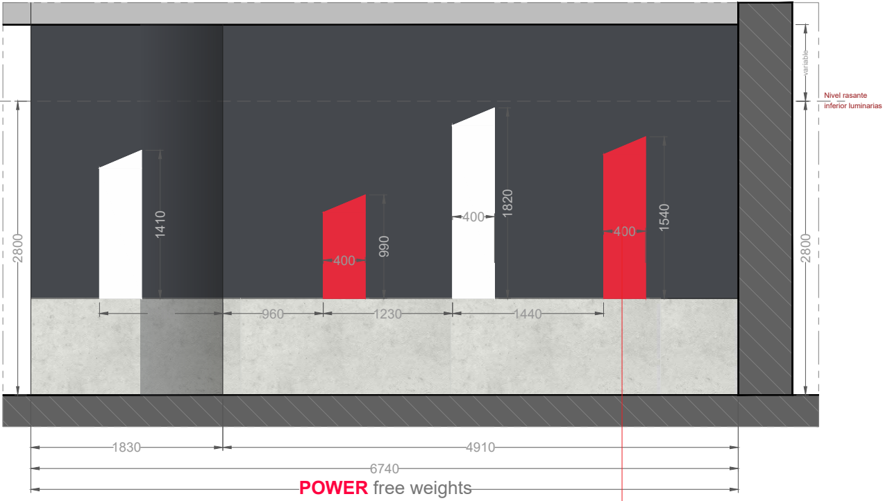
Alzado M | E: 1/50
