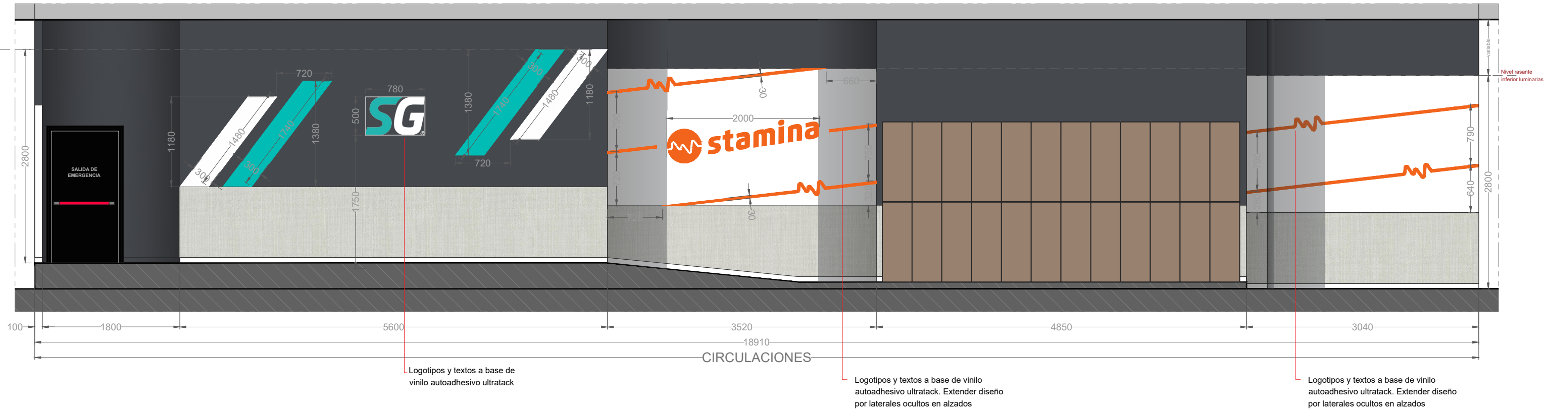
Alzado Z5 | E: 1/50
