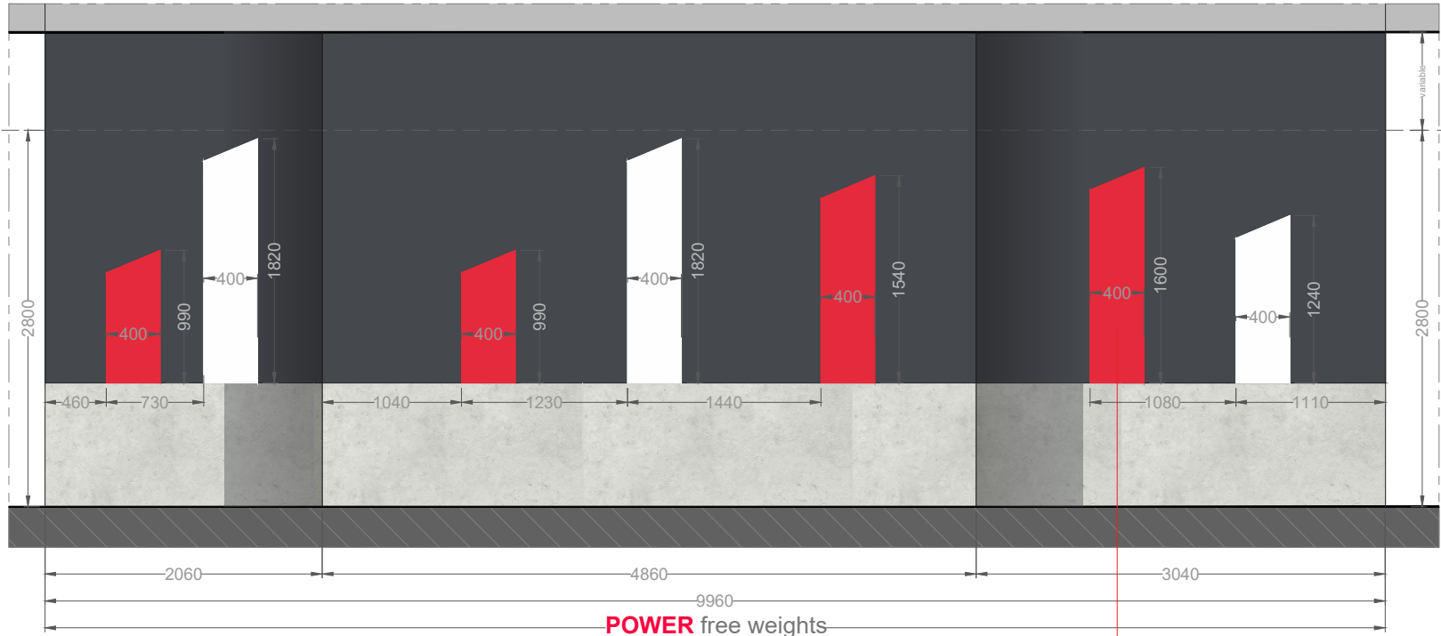
Alzado H | E: 1/50
