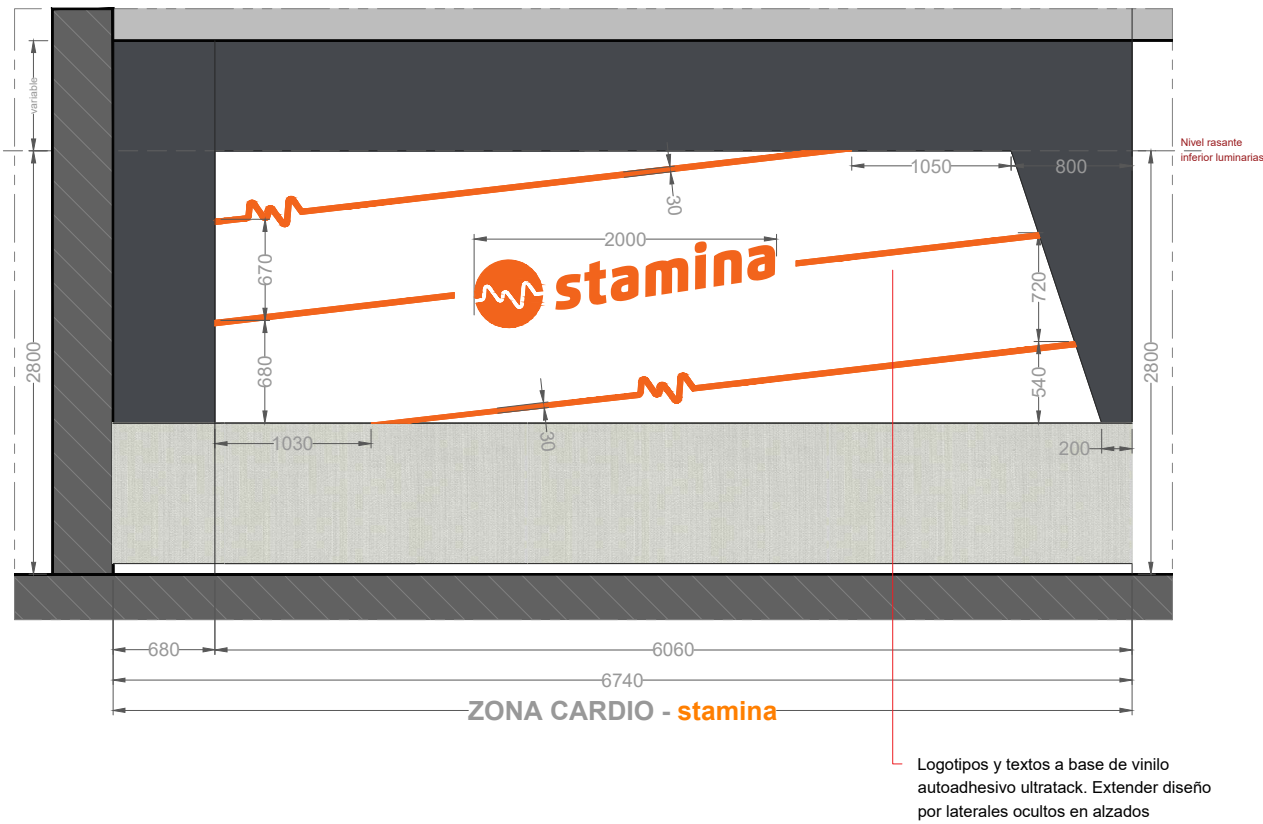
Alzado Z7 | E: 1/50
