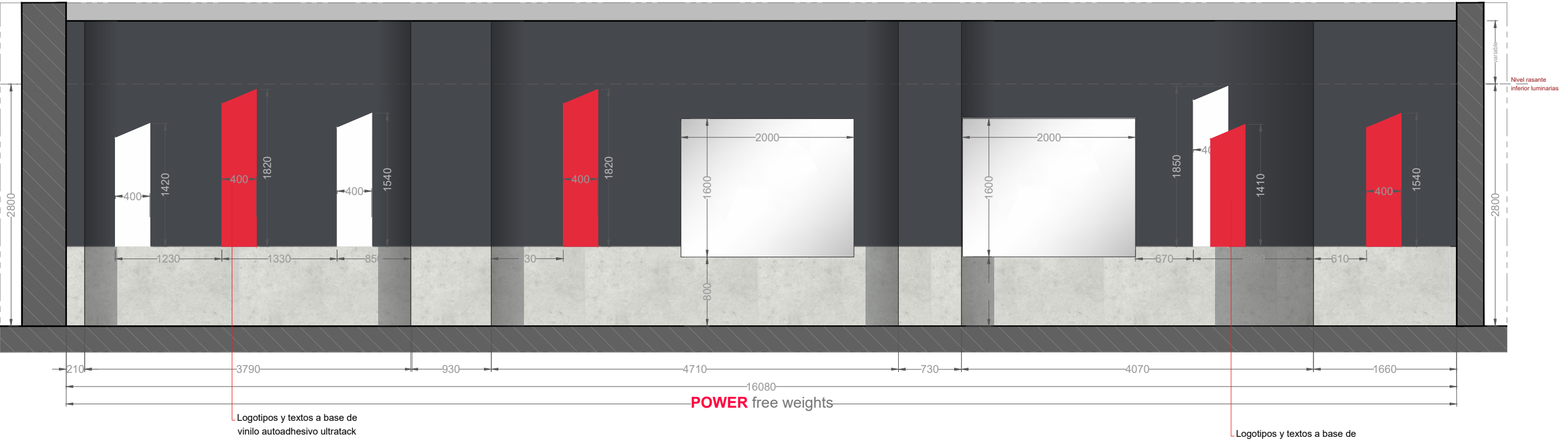
Alzado O | E: 1/50
