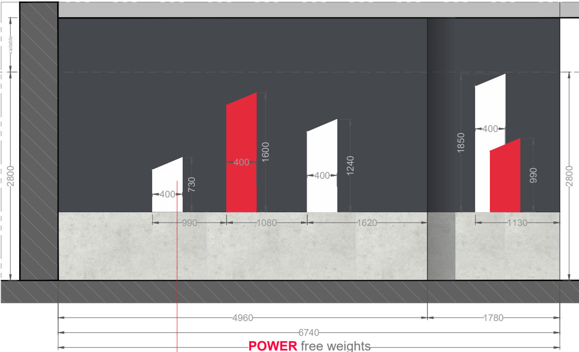
Alzado G | E: 1/50
