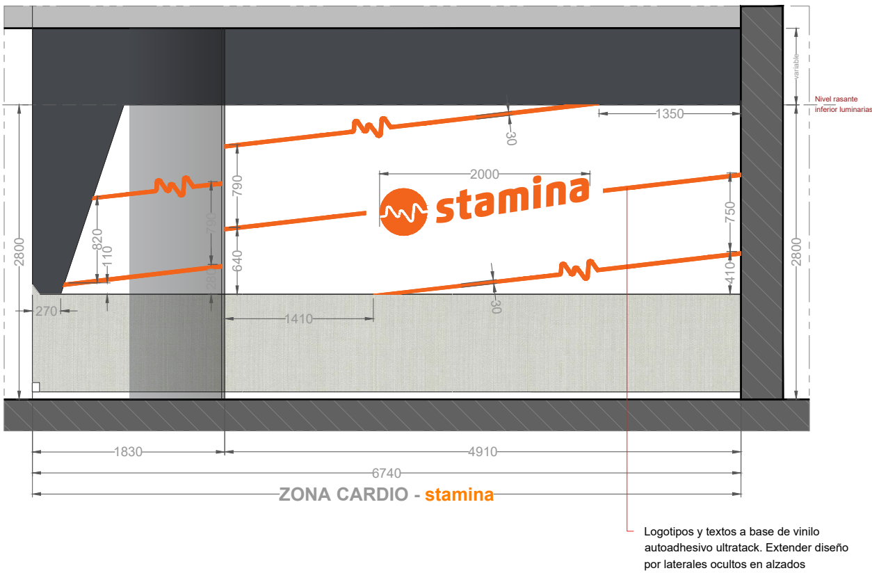
Alzado Z6 | E: 1/50
