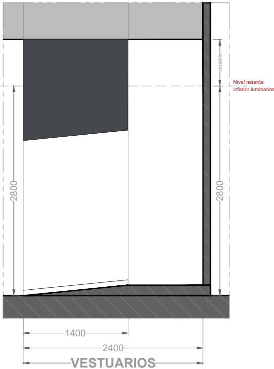
Alzado N | E: 1/50
