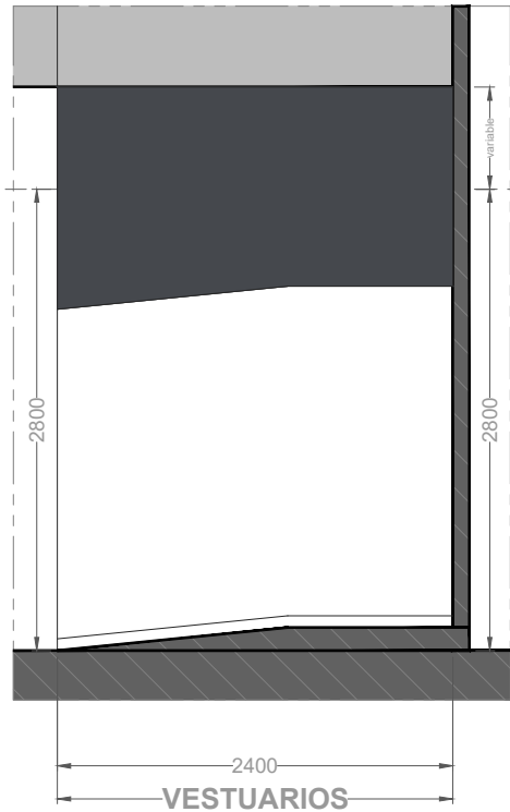
Alzado Q | E: 1/50
