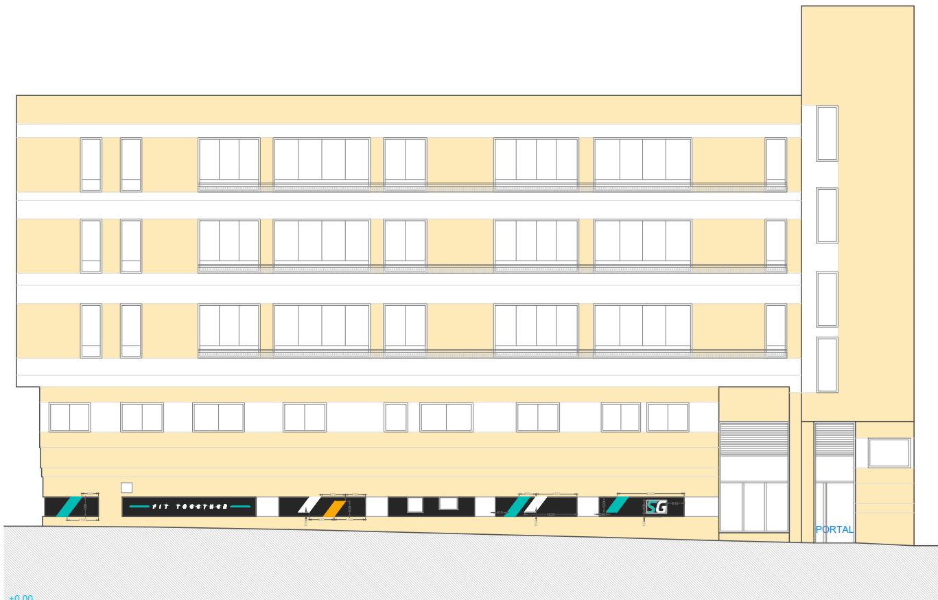
ALZADO 04 CALLE HOLANDA
