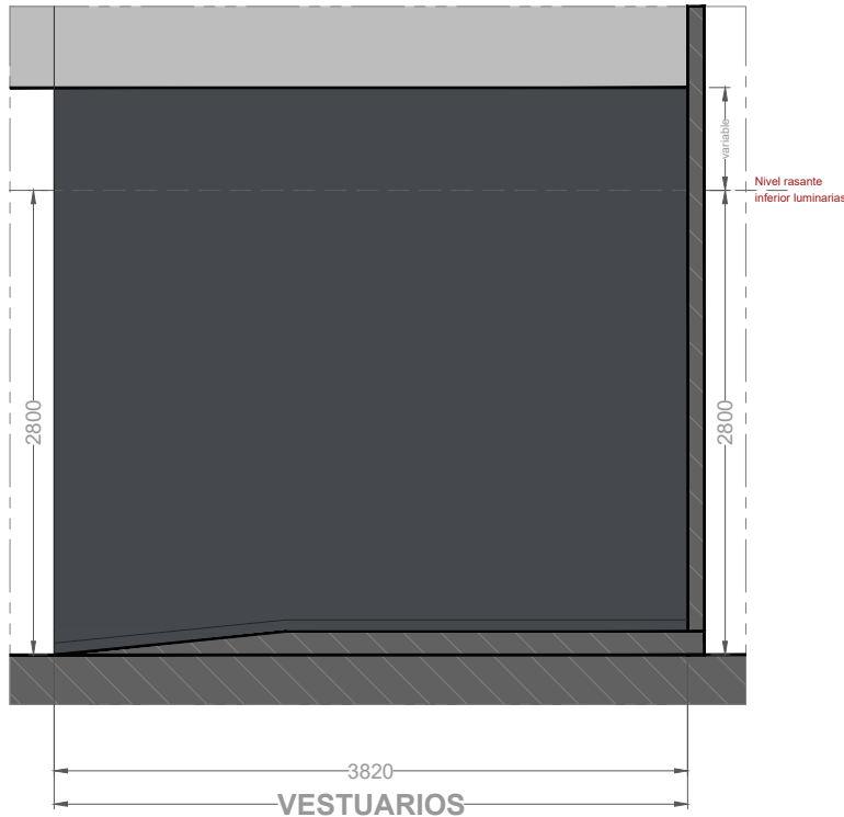
Alzado R | E: 1/50
