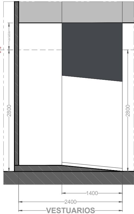
Alzado P | E: 1/50
