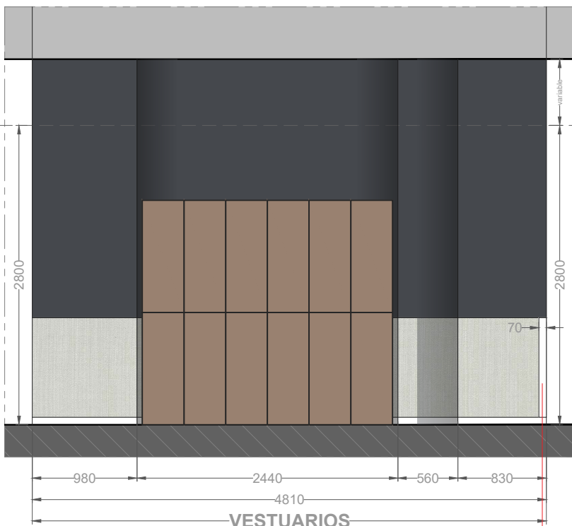
Alzado U | E: 1/50
