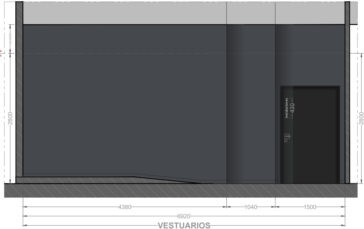
Alzado S | E: 1/50
