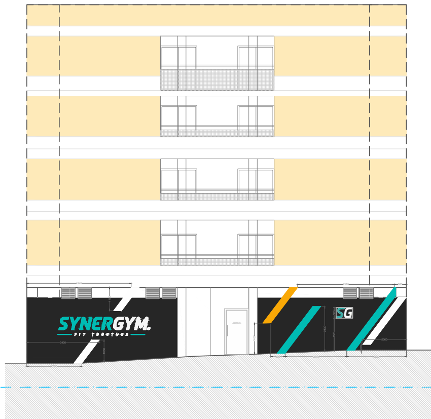
ALZADO 02b CALLE MONTECARMELO 3 - DETALLE ALZADO DESPLEGADO
