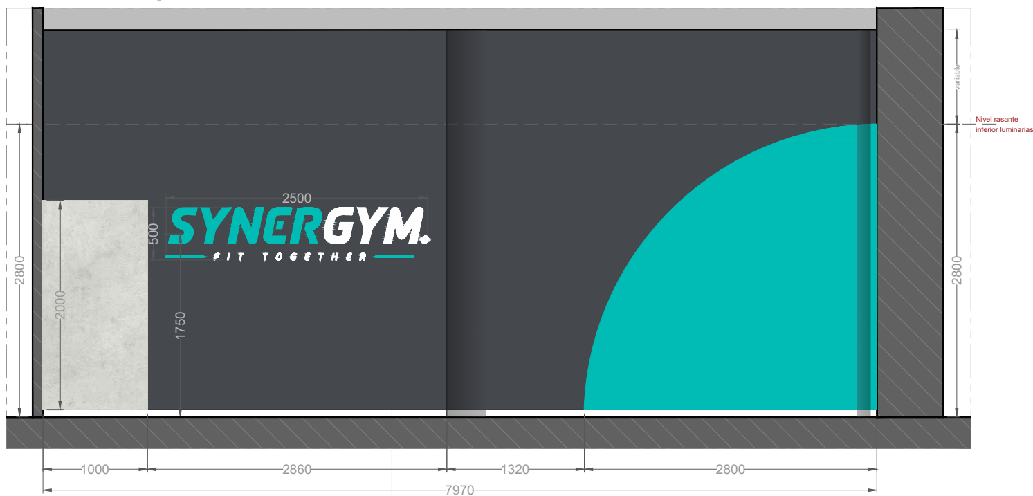
Alzado 2 | E: 1/50
