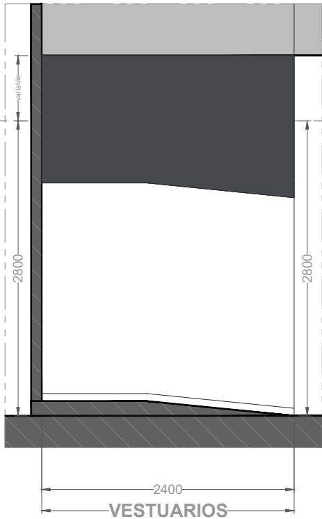
Alzado O | E: 1/50
