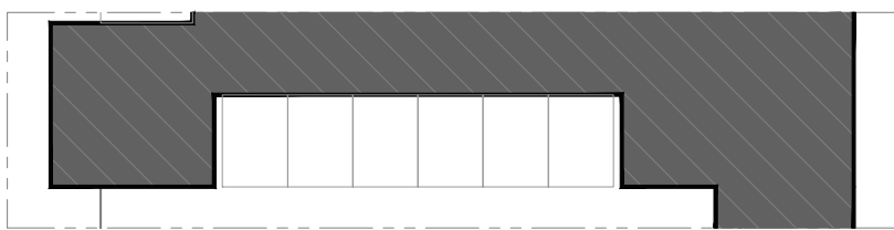
Alzado U | E: 1/50
